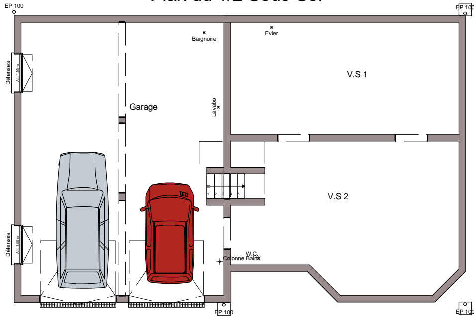
Plan du 1/2 Sous-Sol
